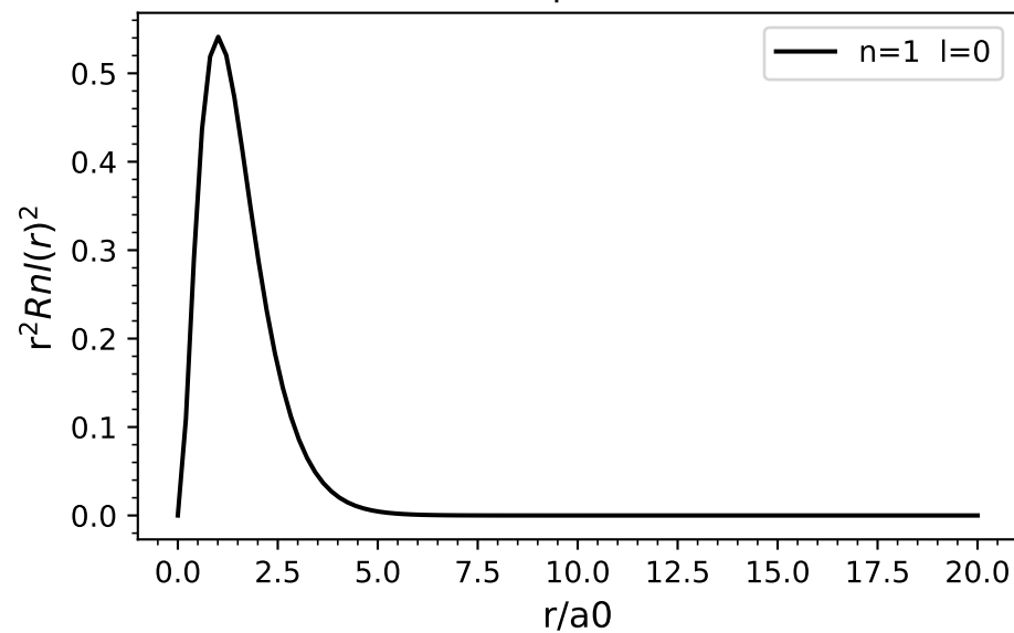
Densité de probabilité P_{nl}
