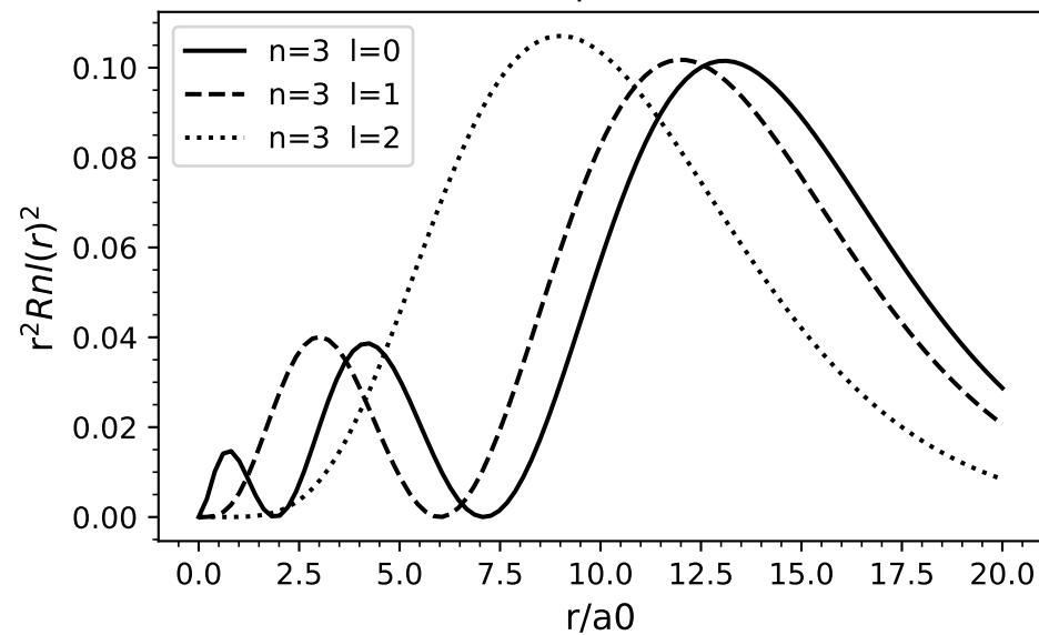
Densité de probabilité P_{nl}
