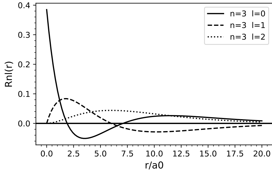
Fonction d'onde radiale R_{nl}(r)
